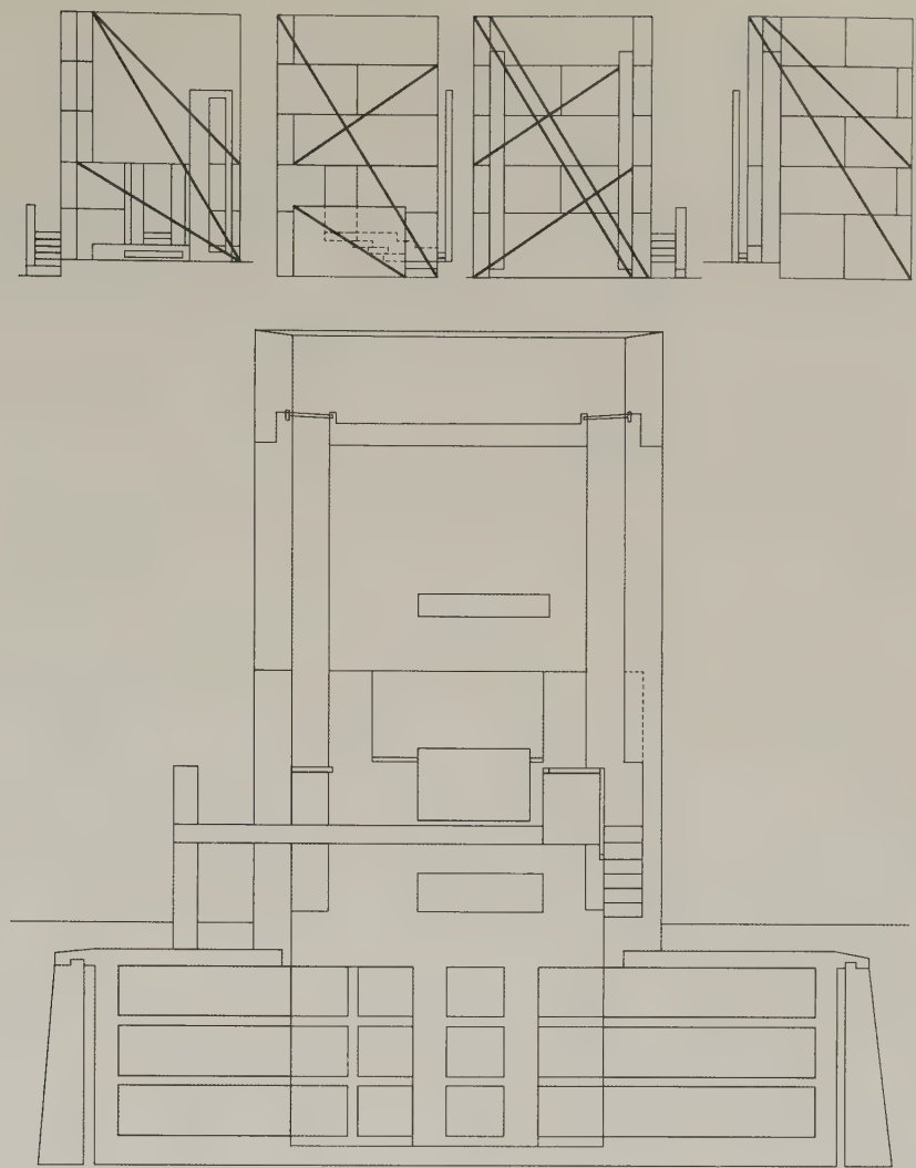
Fig.10 Mambretti Tomb, Fino Mornasco (Giuseppe Terragni, 1938), elevations and transverse section
