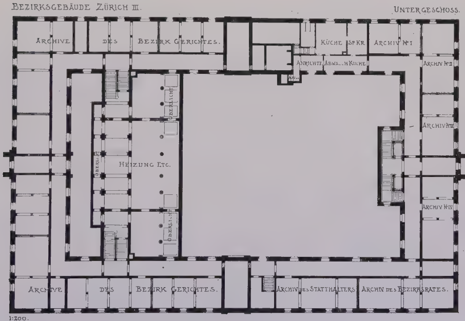
BEZIRKSGEBÄUDE ZÜRICH III.
