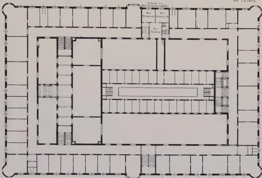
BEZIRKSGEBÄUDE ZÜRICH III.
