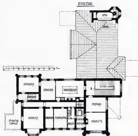
Palais Morozoff, Moskau, F. SCHAECHTEL, Architect, Moskau.
