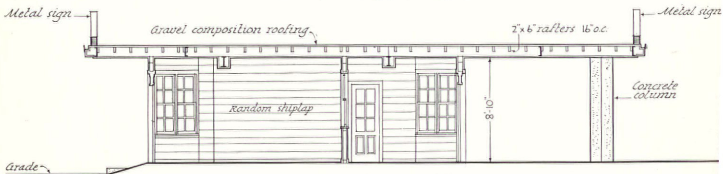
LONGITUDINAL SECTION
