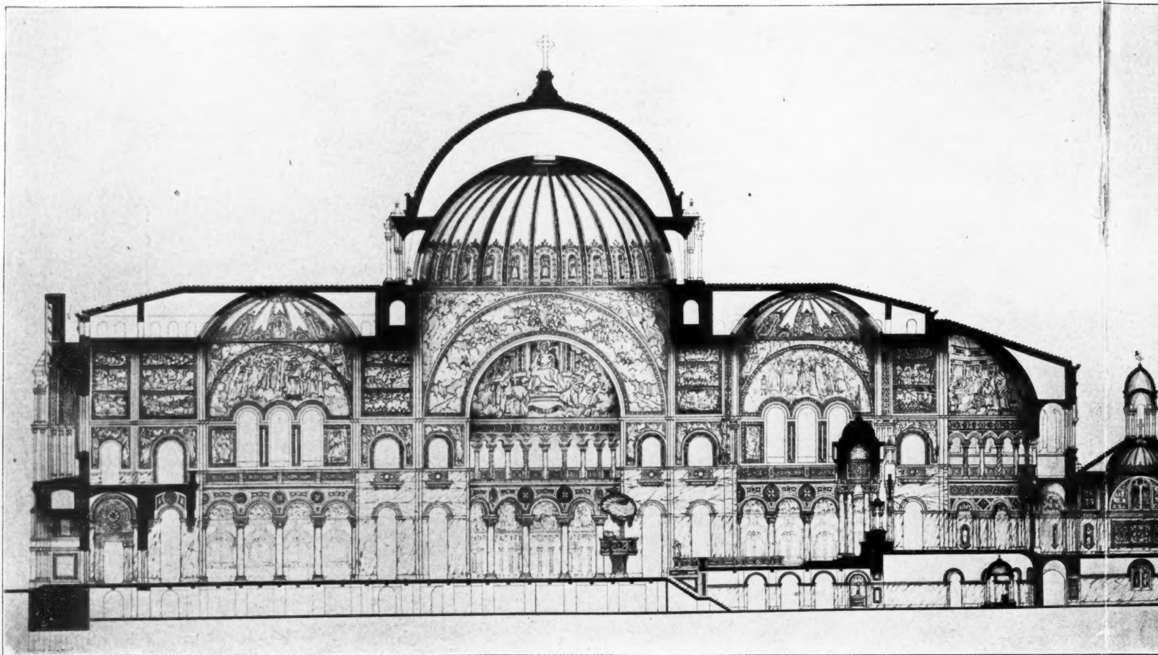
LONGITUDINAL SECTION.
