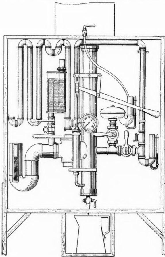
FIG. 24. PNEUMATIC APPARATUS.
