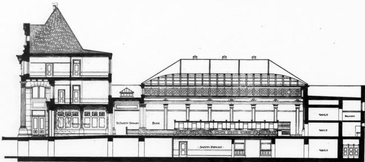
LONGITUDINAL SECTION.
