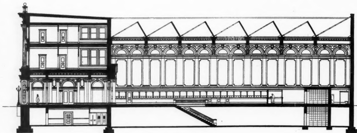
LONGITUDINAL SECTION.
